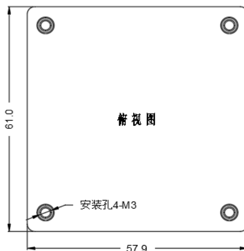
标准型 61.0*57.9*12.7mm
