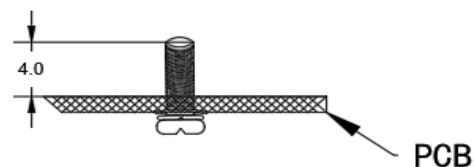
标准型 60.4*39.0*12.7mm
