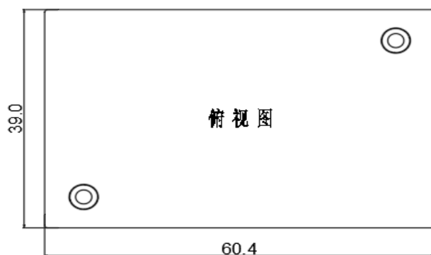
标准型 60.4*39.0*12.7mm
