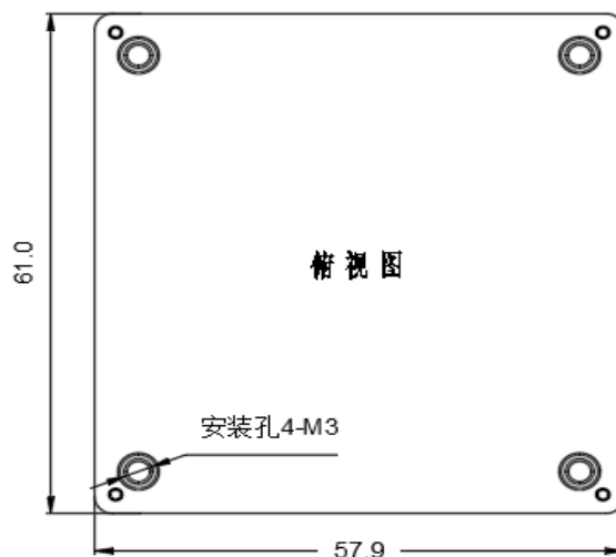
标准型 61.0*57.9*12.7mm
