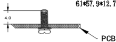
标准型 61*57.9*12.7mm
