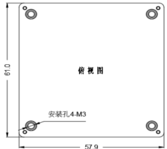
标准型 61*57.9*12.7mm
