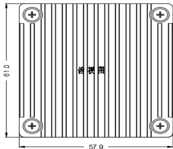
标准型+散热器 61.0*57.9*27.7mm
