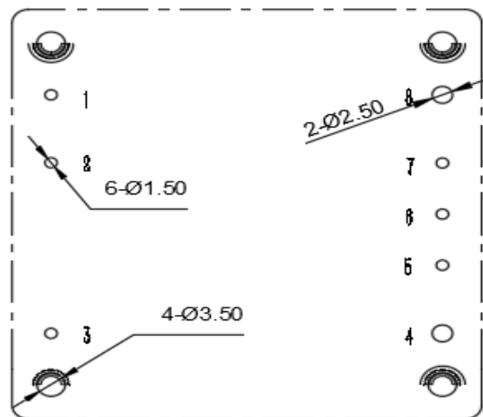
推荐PCB开槽尺寸
