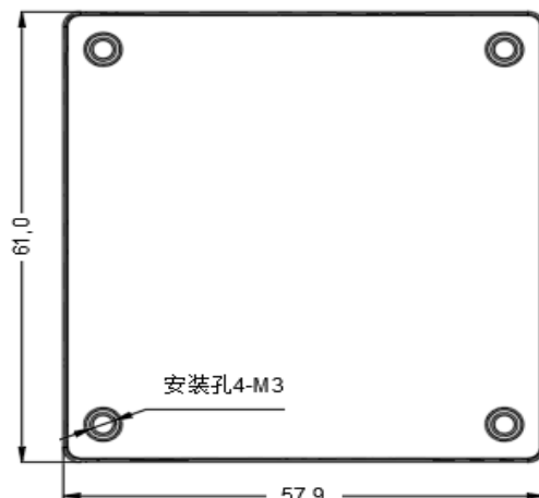
标准型 61.0*57.9*12.7mm
