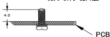
标准型 61.0*57.9*12.7mm
