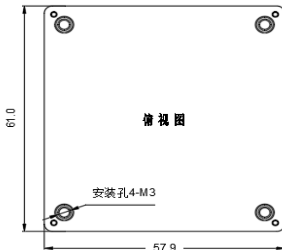
标准型 61.0*57.9*12.7mm
