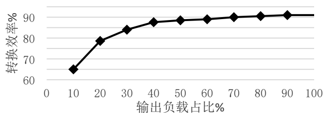
负载效率曲线
