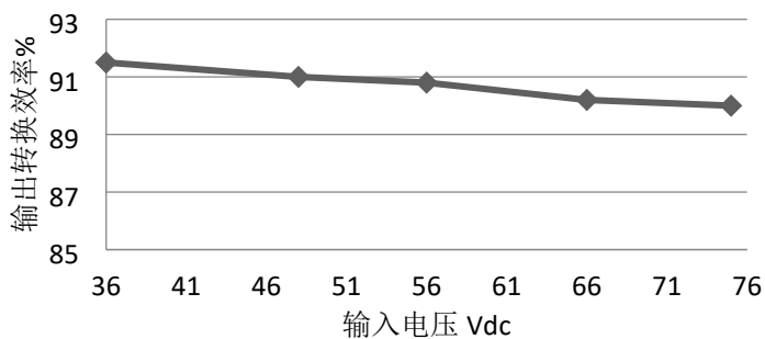
输入电压线性效率曲线
