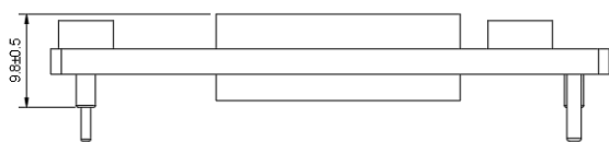
标准型 58.1mm*23.0mm*9.8mm
