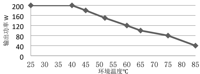
温度降额曲线
