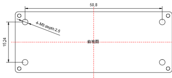
标准型 58.1mm*23.0mm*9.8mm
