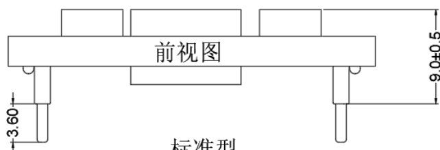
标准型 34. 3*24. 1*9. 0mm
